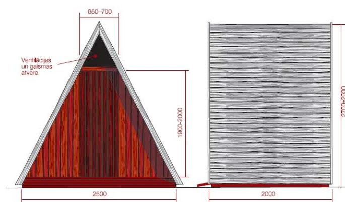
Pretskats un sānskats
